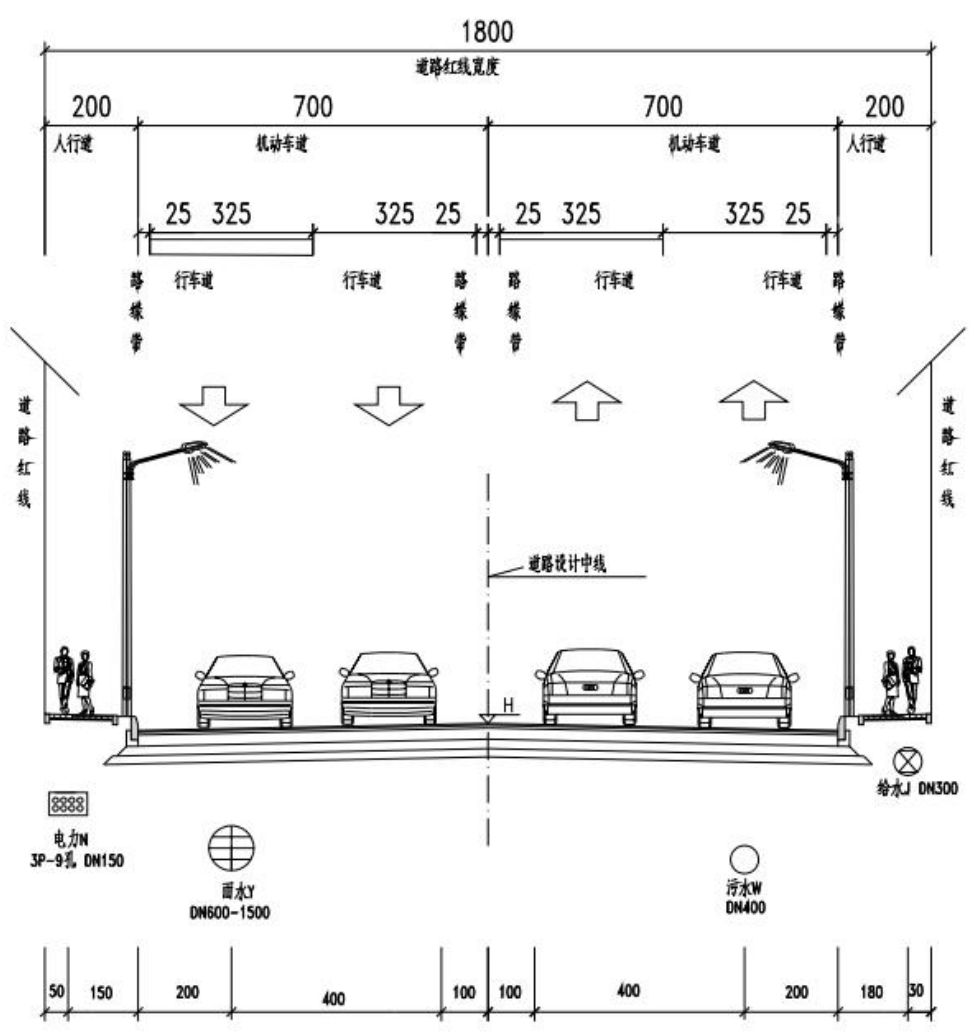
图 4-6 管网标准横断面图
