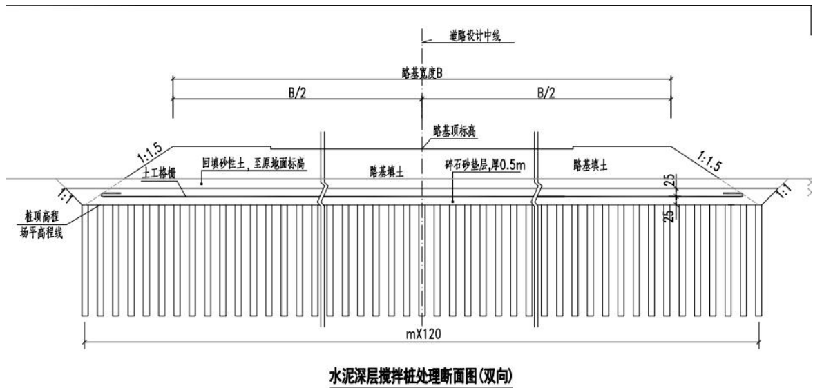
图 4-4 水泥深层搅拌桩处理断面图（双向）
