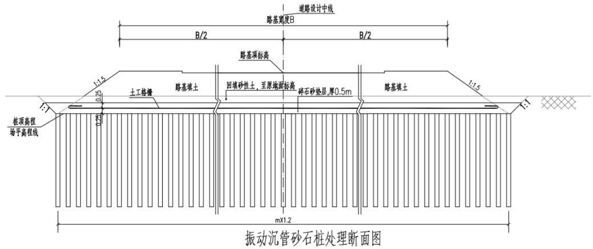
图 4-5 震动沉管砂桩处理断面图
