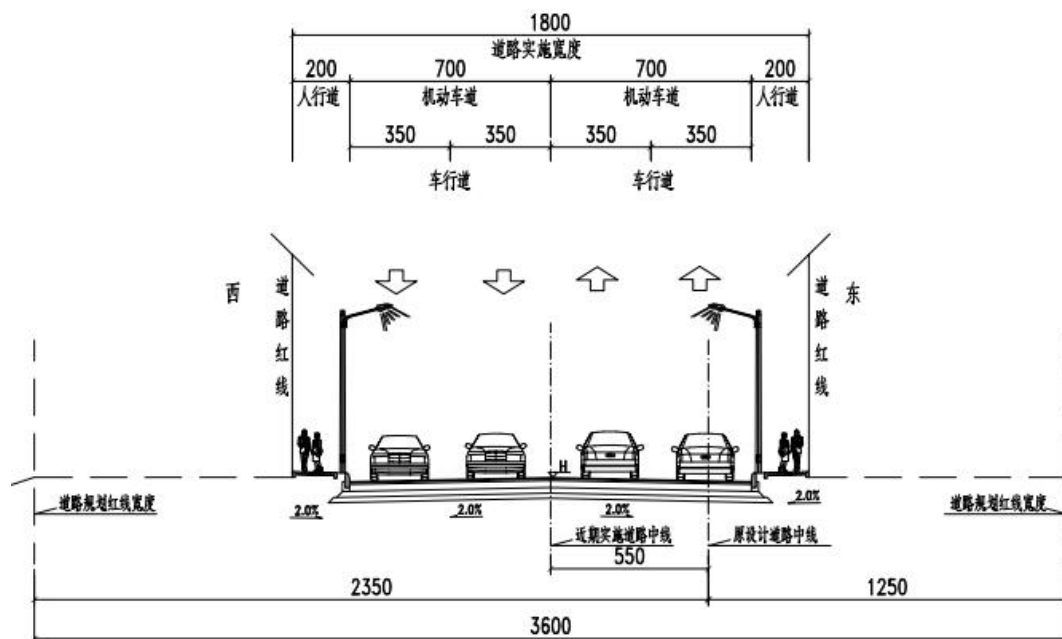
图 4-2 道路横断面
