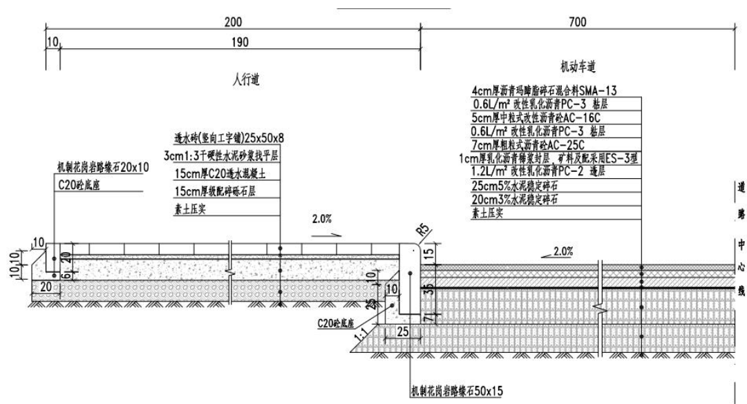
图 4-3 路面结构图
